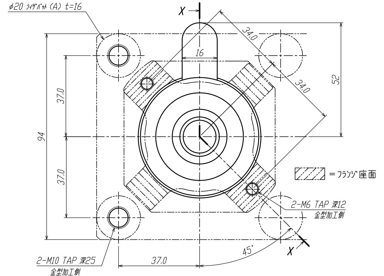
寸法表 1 (ノズル温度250℃のとき)
