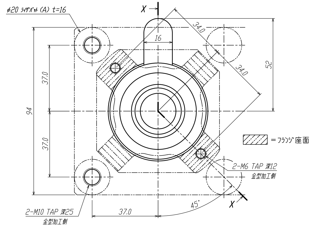
図1 寸法表 (ノズル温度250℃のとき)
